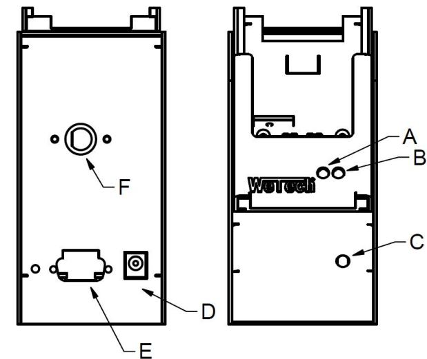
Schemazeichnung DP1-669USB
